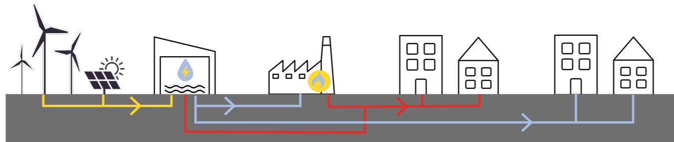
Waterstofproductie en levering aan gebouwen via warmtenet (rood) met restwarmte en/of centraal stookhuis, danwel rechtstreeks als gas aan gebouwen
