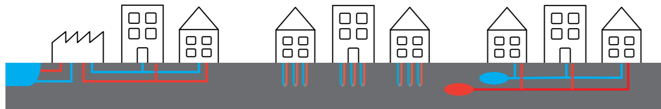
Warmte en koude-opslag in de bodem. Midden met een individueel gesloten WKO-systeem. Rechts met open WKO en een bronnet (laag temperatuur warmte- en koudenetwerk). In plaats van een open WKO is een bufferopslag ook een optie. Bij aquathermie (links) wordt uit oppervlaktewater of rioolwater warmte/koude afgevangen en op een warmte/koudenet gezet.
